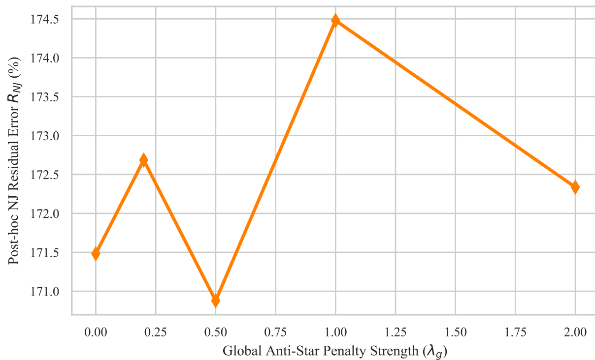
(D) Phase 3 Macro-Topological Invariance
